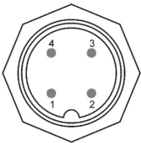
Abb. 2 Elektrischer Anschluss
