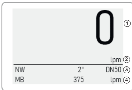
Abb. 6: Display Startansicht
