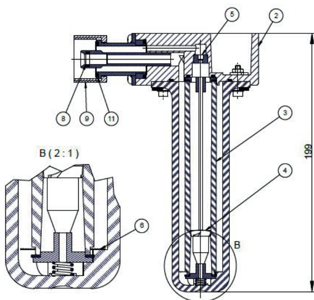
Abb. 2: Positionszeichnung Nebenstrommessgerät
