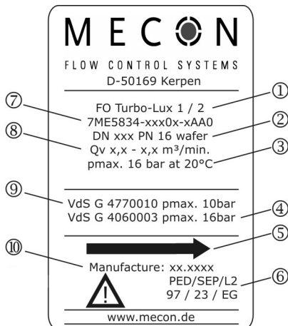
Abb. 2 Typenschild Messblende
