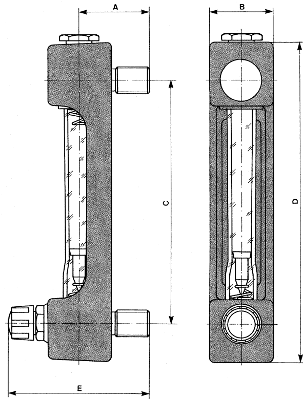
Рисунок 3 Minix, размеры
