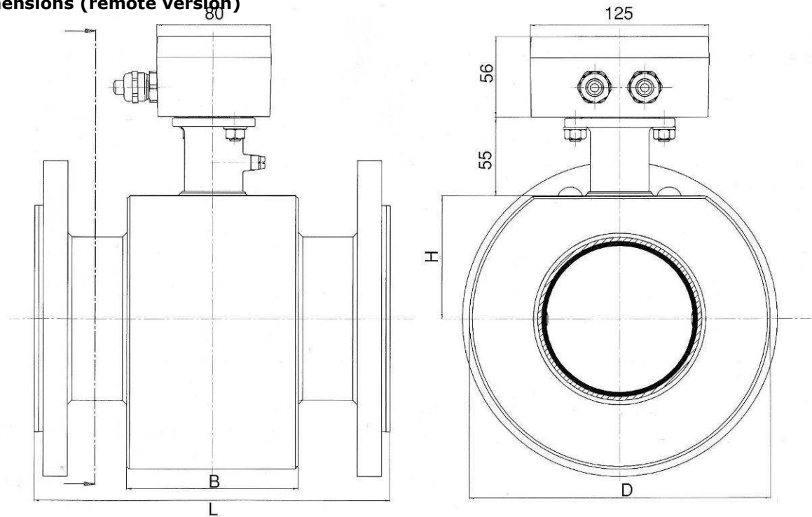
Fig. 10 Dimensions
