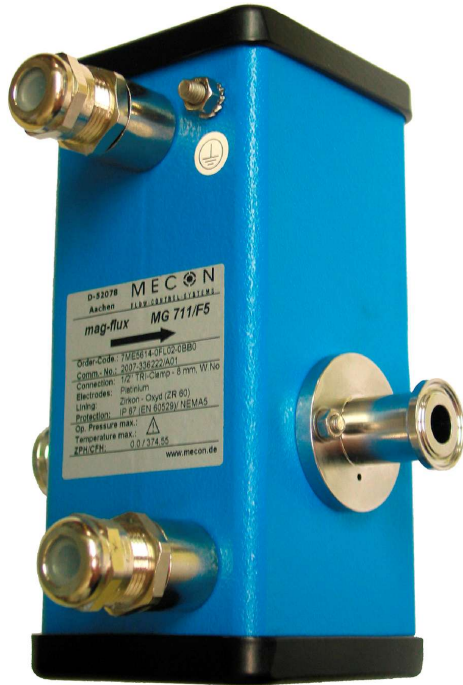
Bild 1 Magnetisch Induktiver Durchfluss Sensor mag-flux F5
